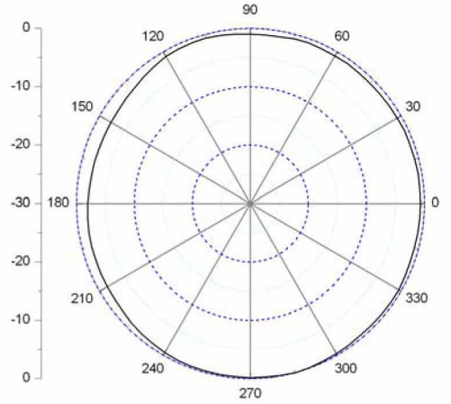
E-Plane
