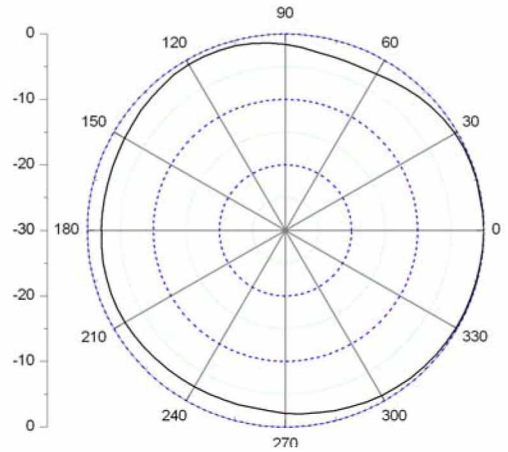
E-Plane
